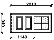
TYPE D1.1 1 stk 94x201 cm INDDØJENDE HH MED 10X50 MM SKINNE ISTEDET FOR BUNDSTYKKE SNYDESPROSSER FOR RUDE
